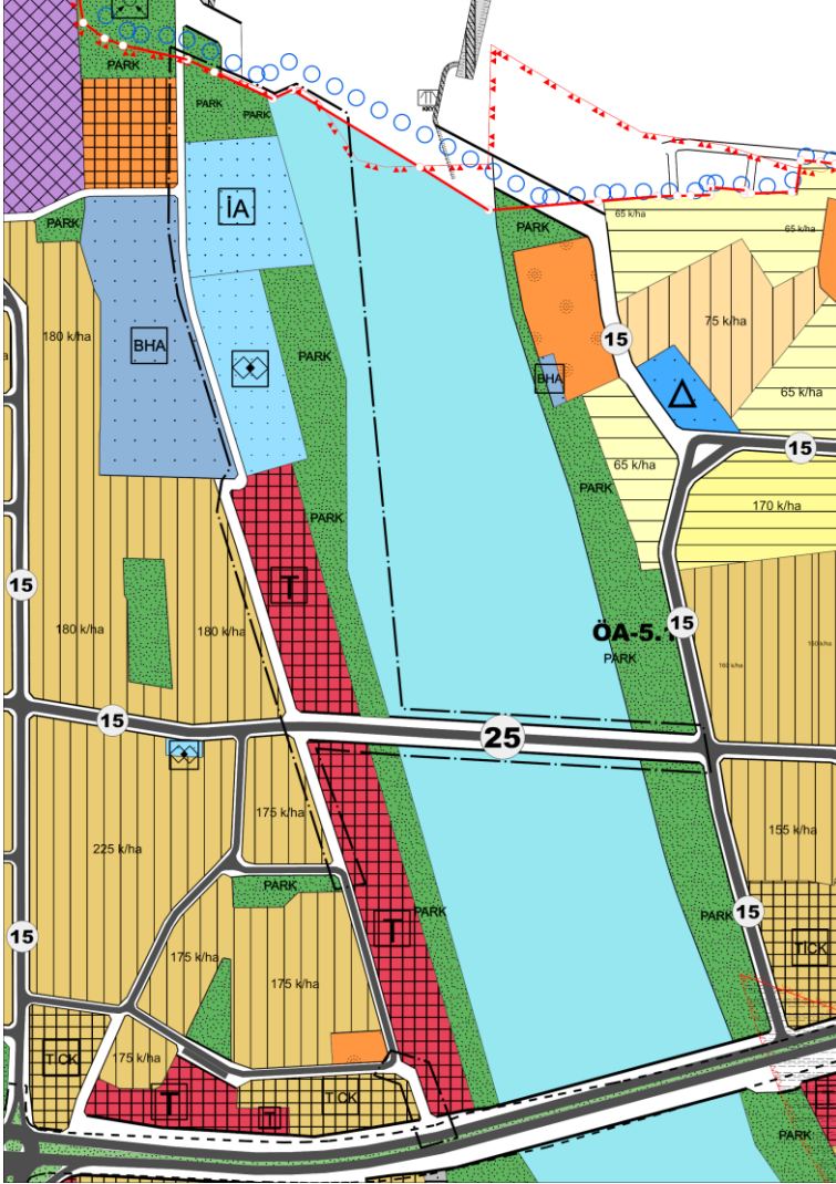
MEVCUT NAZİM İMAR PLANI
