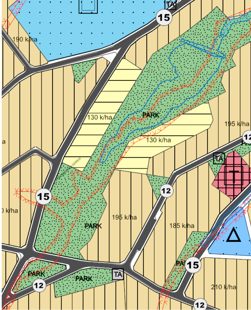
MEVCUT NAZIM İMAR PLANI
