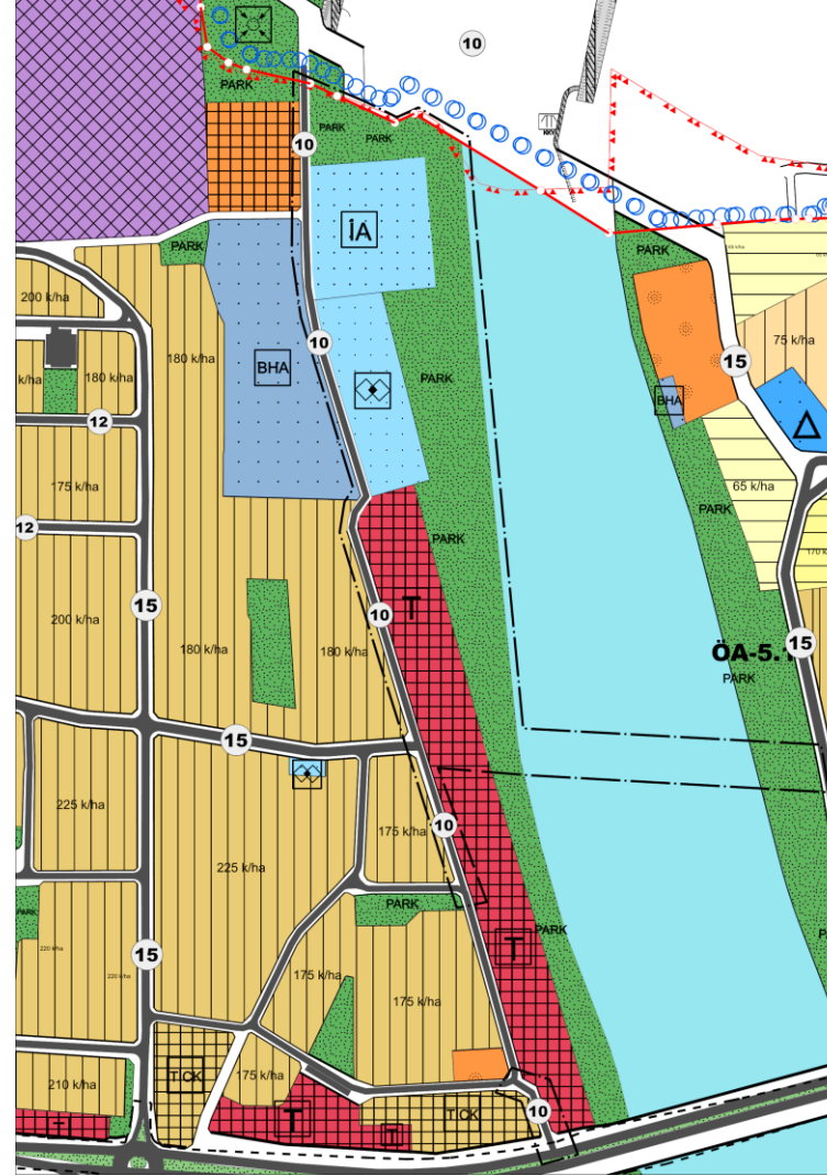
ÖNERİ NAZİM İMAR PLANI
